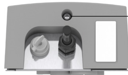
Schraube Unterseite Torx TX25
