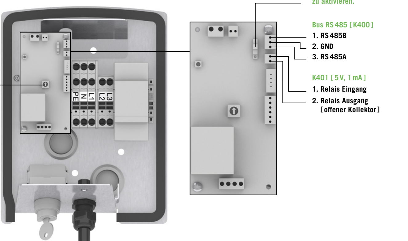
Abbildung 9 Bus-Schnittstelle
